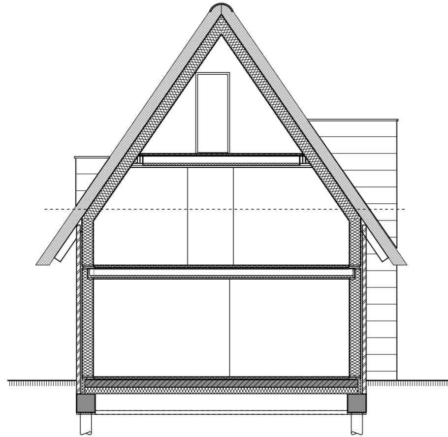
DOORSNEDE A-A
