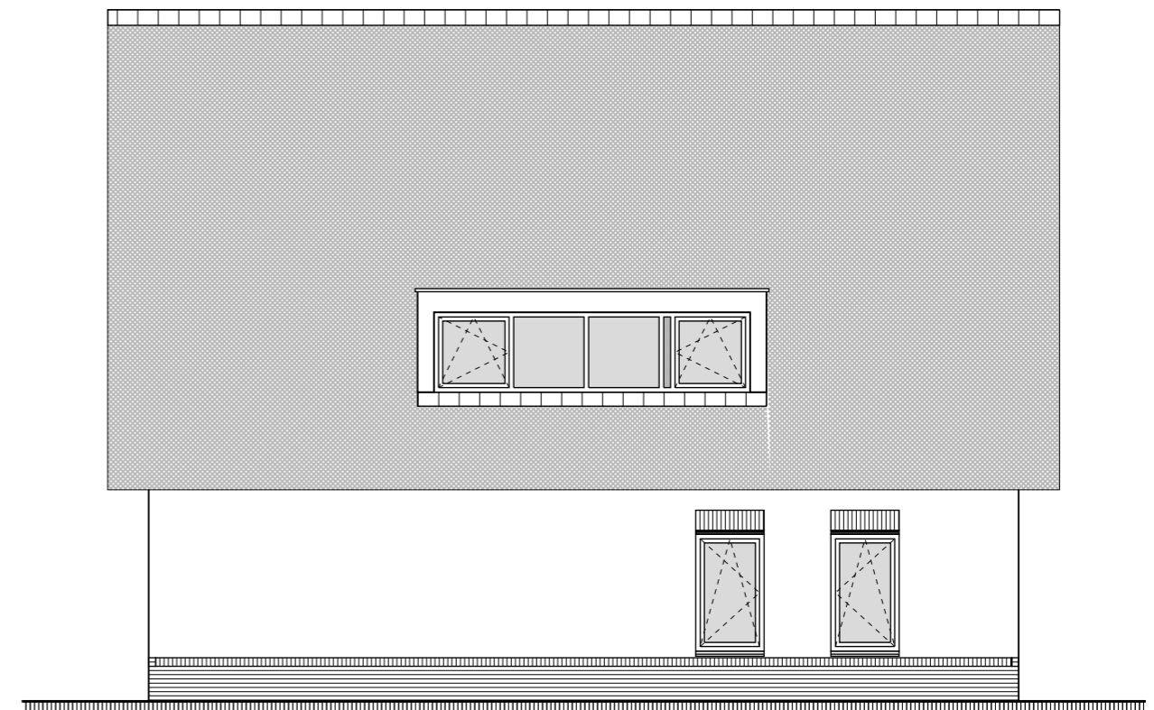
ZIJGEVEL ENTREE
