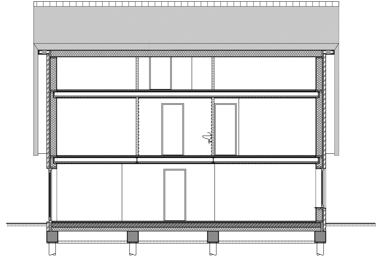
DOORSNEDE B-B
