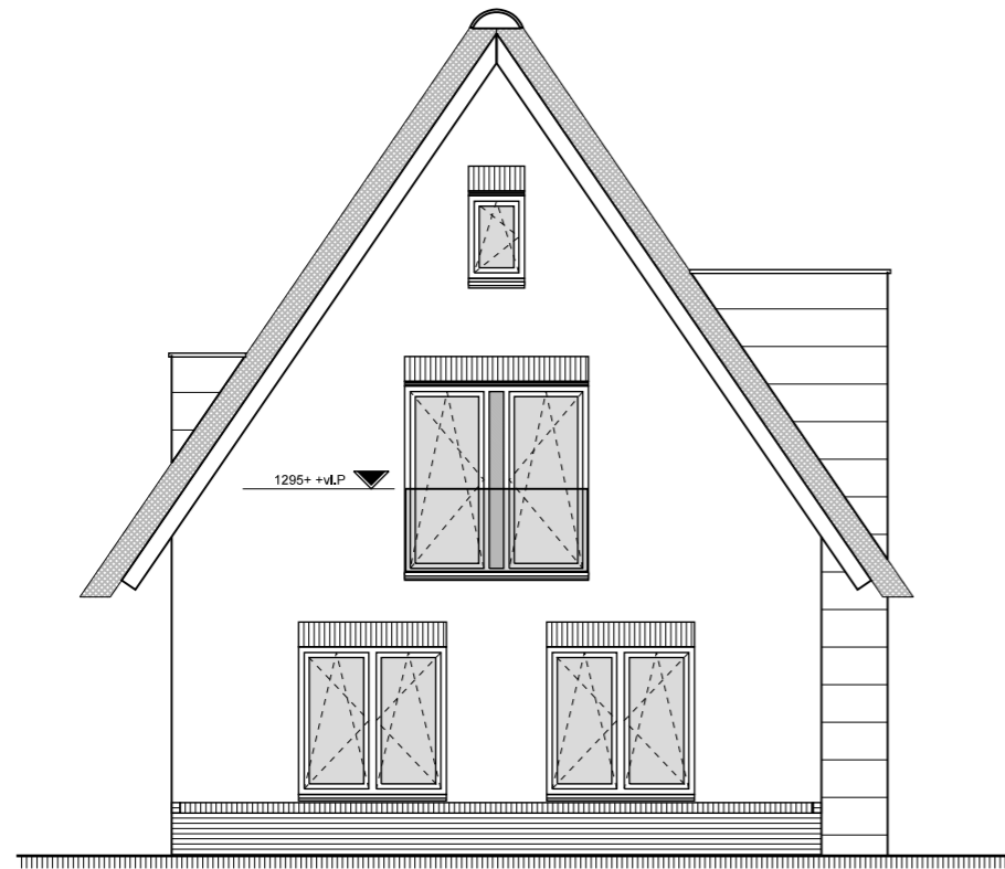
VOORGEVEL
